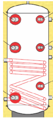
Τύπος COS-1P
